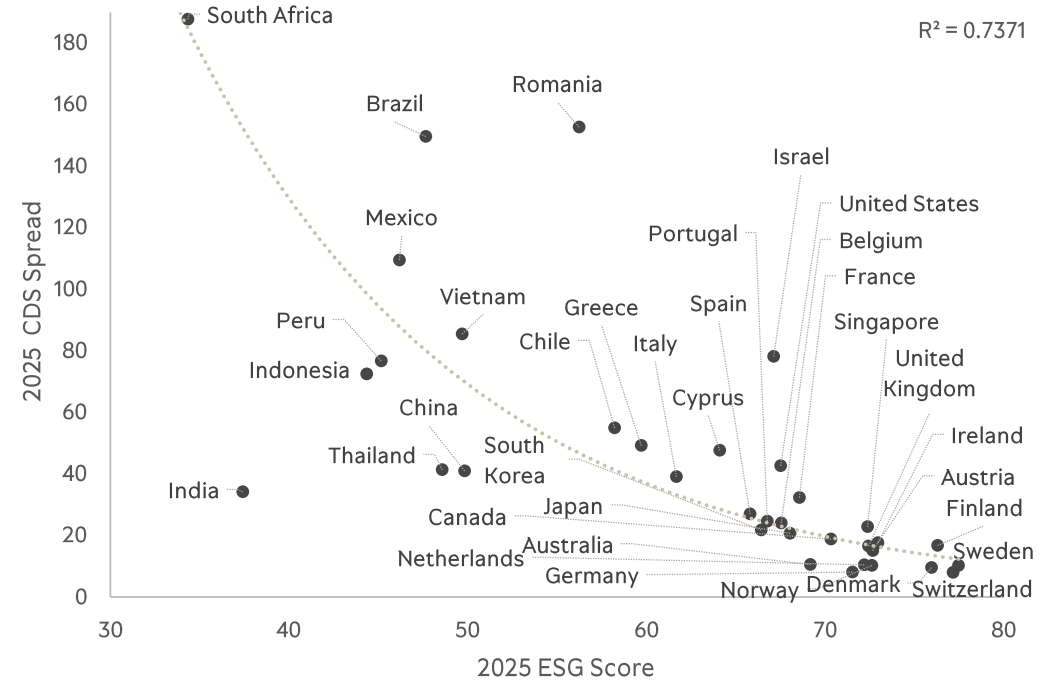
Valuation & Sovereign ESG Score
